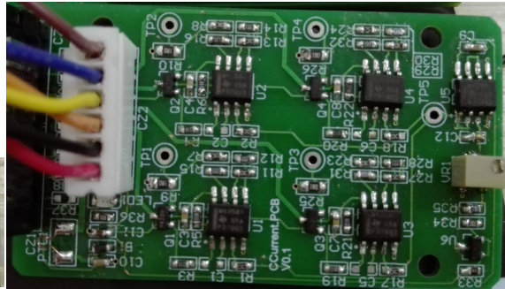
控制板
