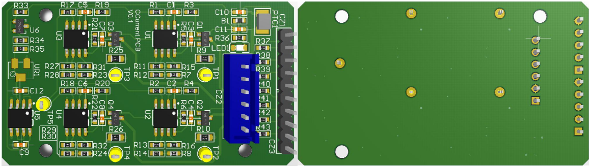
PCB 元件面
